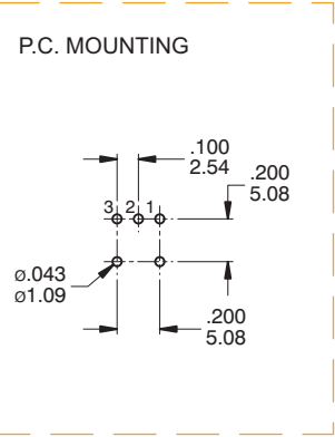
A1, A3 FOR SPDT / A2 FOR DPDT
